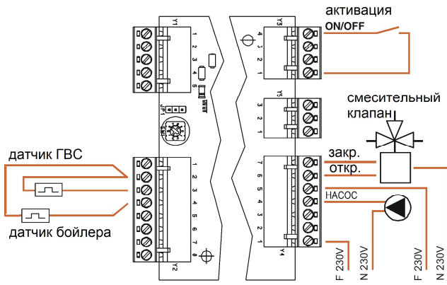
Бойлер ГВС 2
