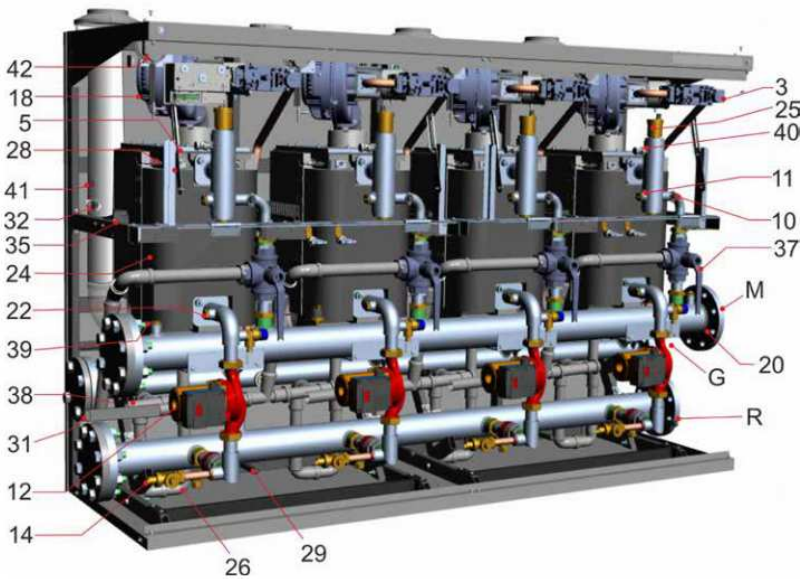
KASKAD 460
