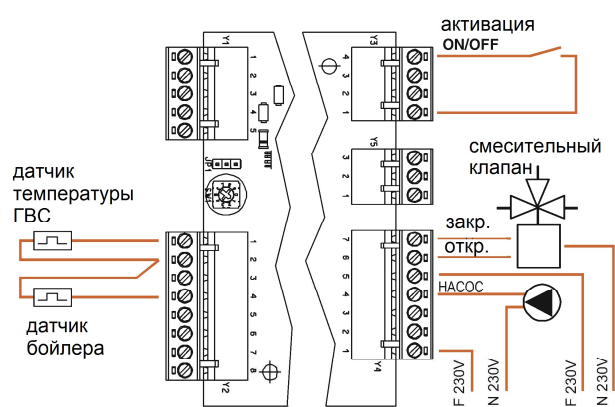
Бойлер ГВС 1
