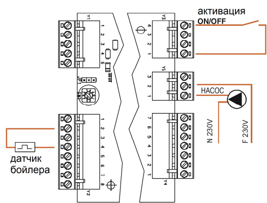
Бойлер ГВС 3
