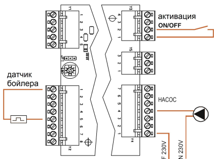
Бойлер ГВС 2
