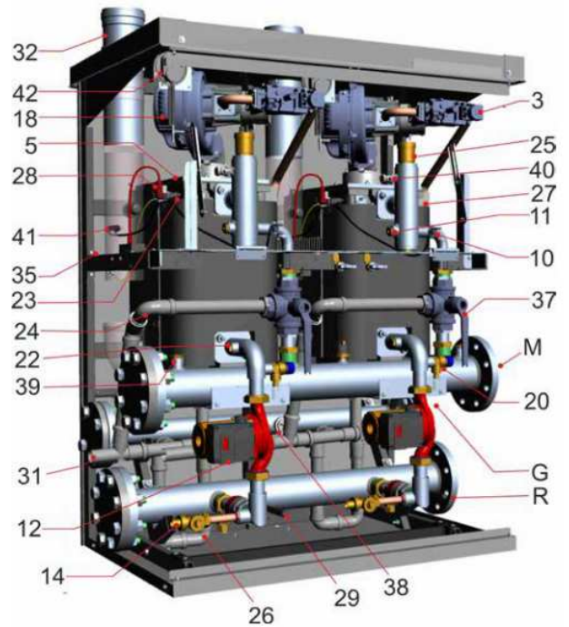
KASKAD 230
