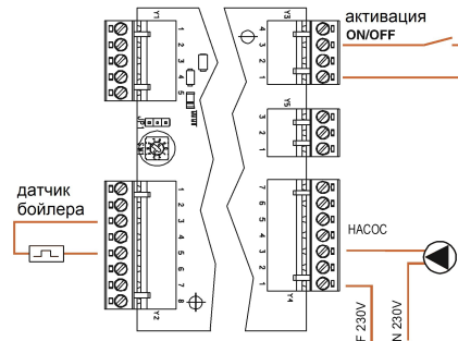
Бойлер ГВС 3
